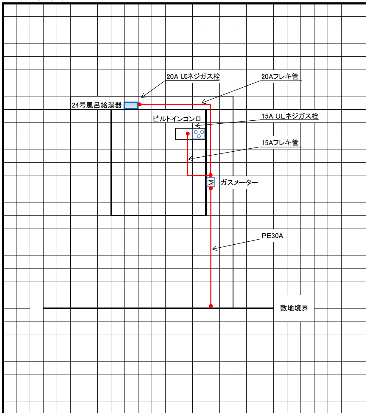
<内管工事の標準モデル図>
